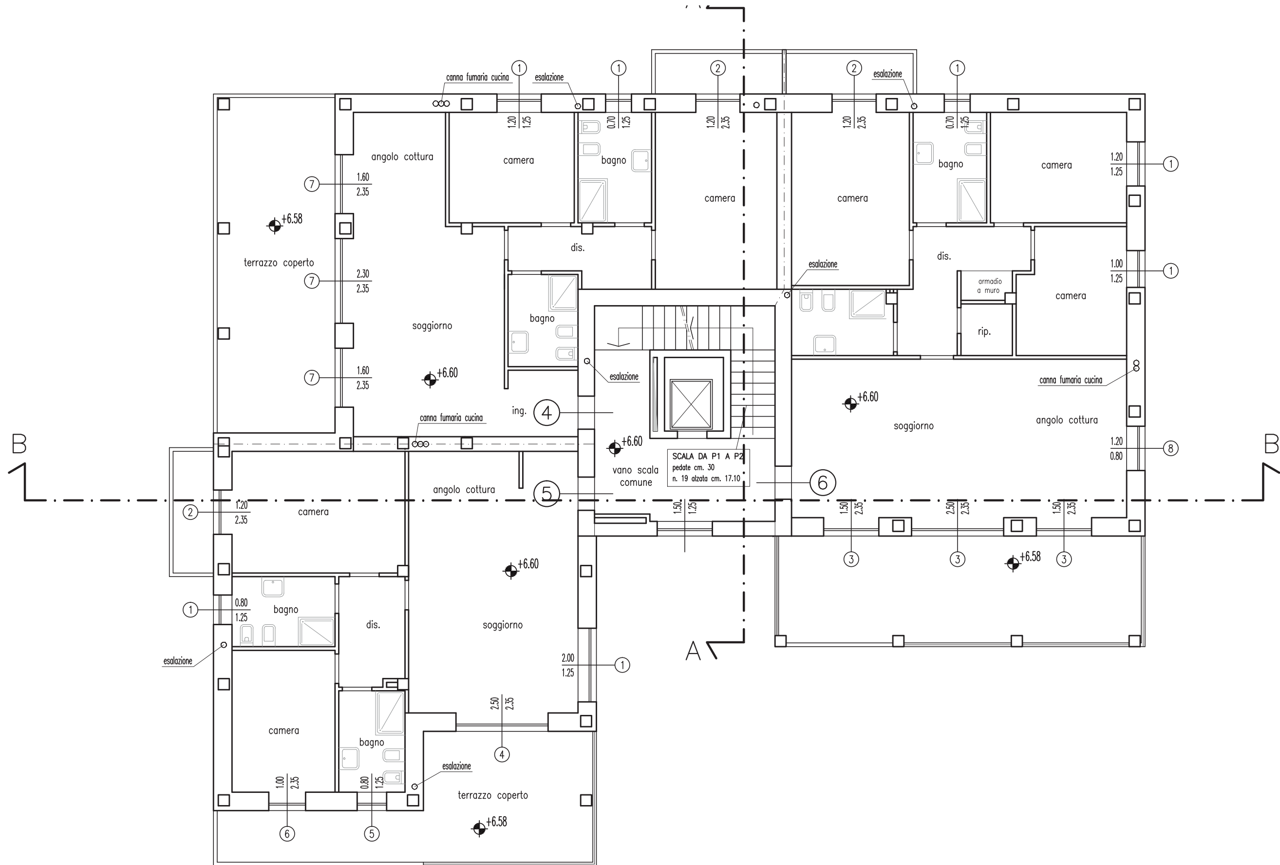
PIANO SECONDO
